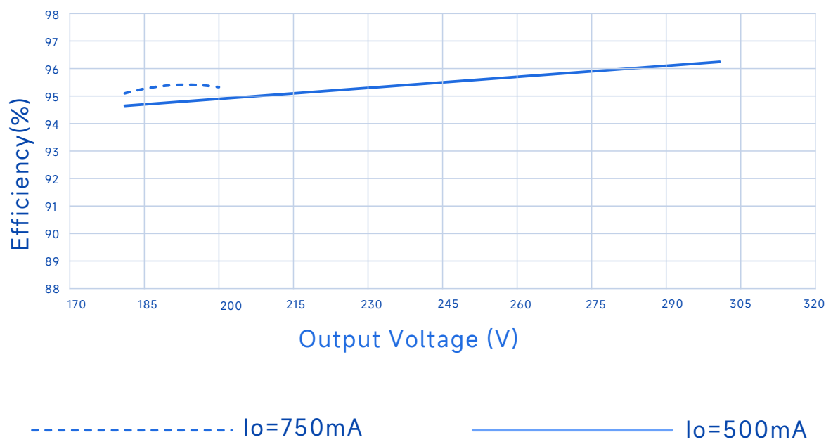
效率 Vs. 输出电压 (Vin=347Vac)
